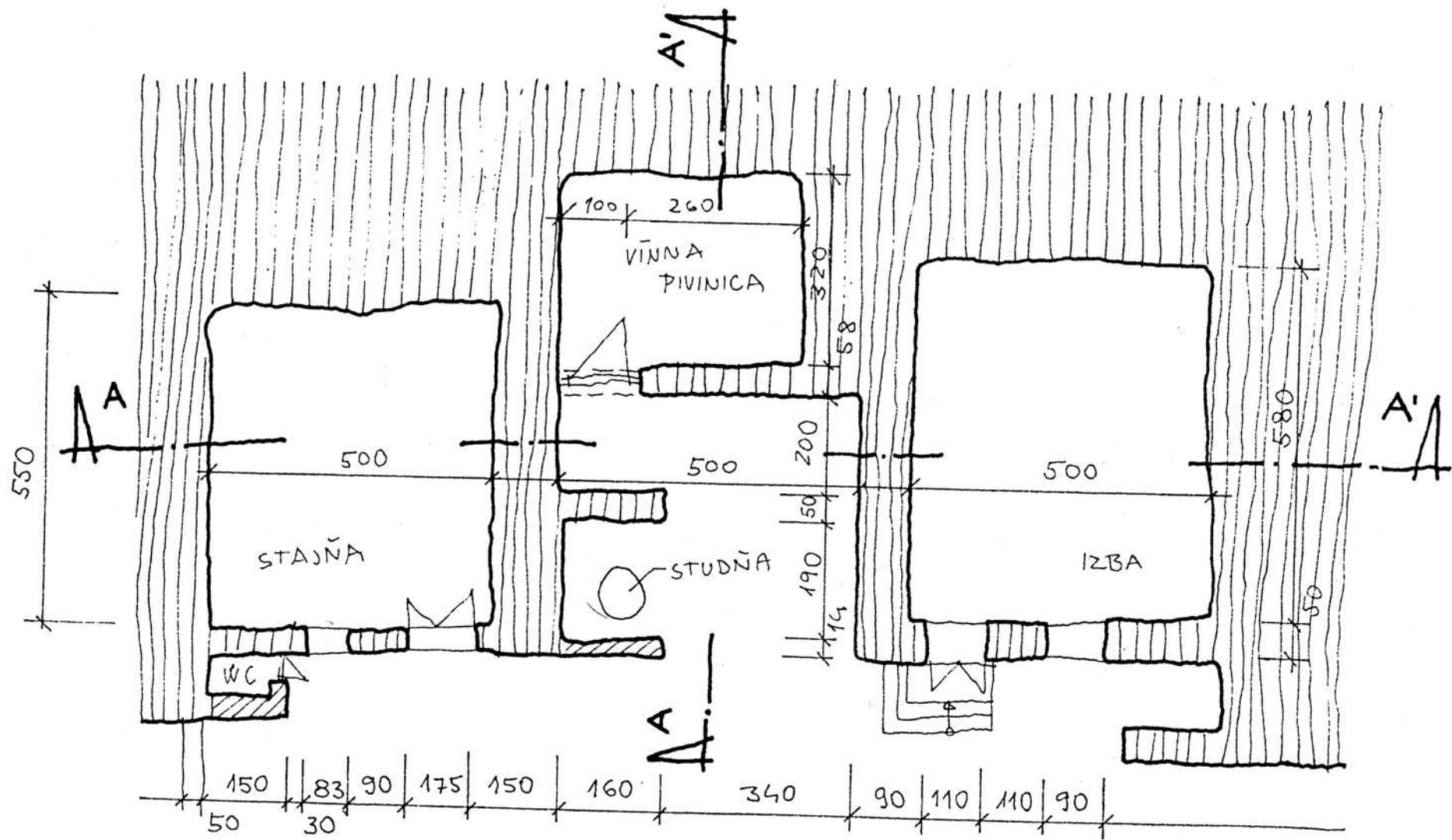
Pôdorys
