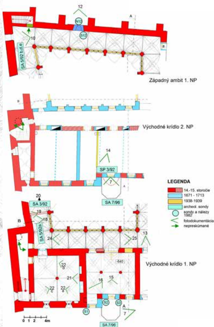
Tab II. Levoča, kláštor minoritov, details pôdorysu krížovej chodby s analýzou stavebného vývoja. Podľa: URBANOVÁ 2015, ref. 2.
