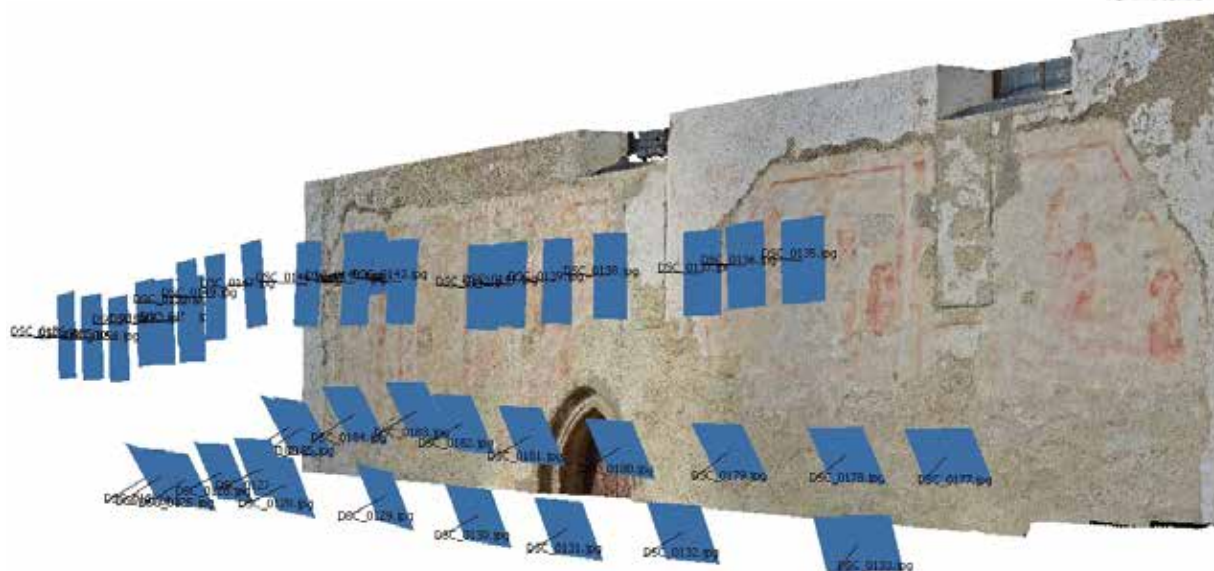
5. Schéma spôsobu snímkovania a výsledná podoba 3D modelu snímanej časti fasády. Autor: M. Marčiš, 2016.
