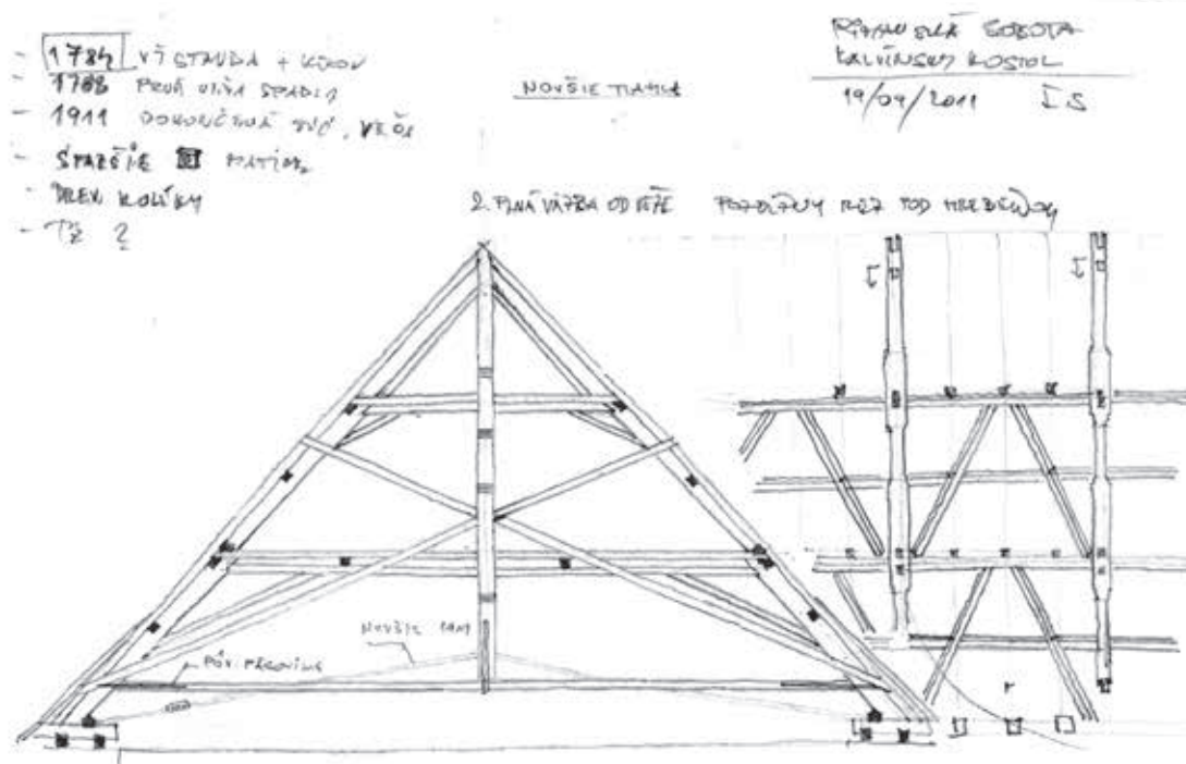
31. Rimavská Sobota, ev. a. v. kostol. Rezy krovom s ležatou stolicou, terénna skica. Autor: Ľ. Suchý, 2011.
