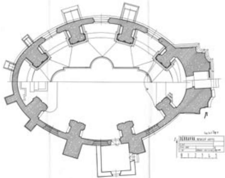
Pútnický kostol v Bratislave - Dúbravke, 1950-51, sign. V 5396
