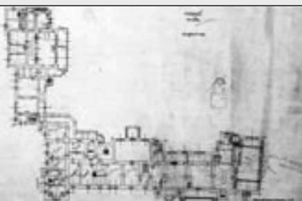
Kaštieľ v Parchovanoch, pôdorys prízemí
