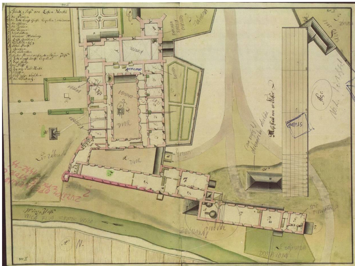
Pôdorys druhého nadzemného podlažia kláštorného areálu (horná časť obrázku - kláštorný kostol, konvent, dolná časť - sýpka, kuchyňa, konvikt, škola, pivovar), rok 1791 ?, MOL No. 116/1-3
