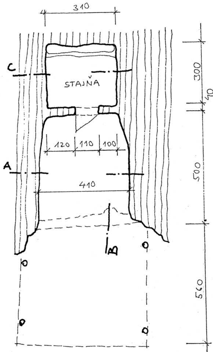
Pôdorys
