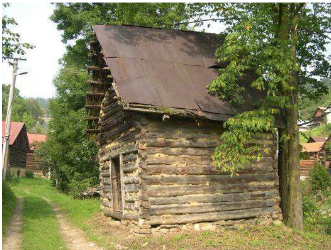
Obr. 85 a 86 – usadlosť č. 26 – zrubový sypanec + detail konštrukcie zrubu
